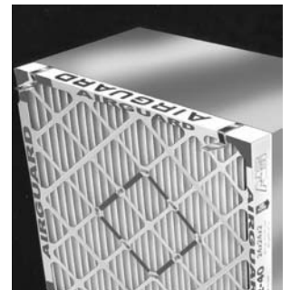
Filtro plisado de 2" tipo DP montado en el frente de un filtro de caja rígida Vari-Pak con un adaptador de prefiltro RC-79-1.
